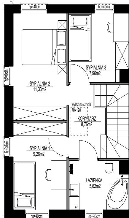
RZUT PIĘTRA
