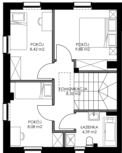
RZUT PIĘTRA
