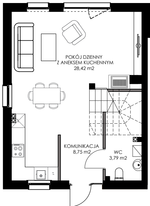
RZUT PARTERU
