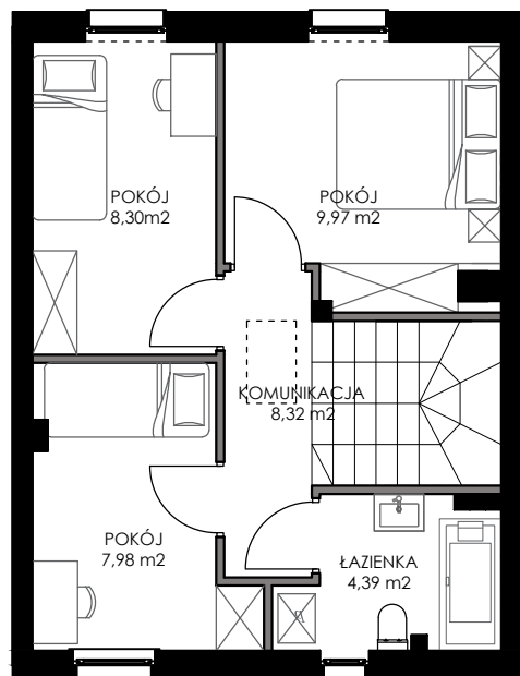
RZUT PIĘTRA
