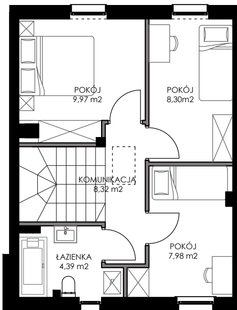
RZUT PIĘTRA
