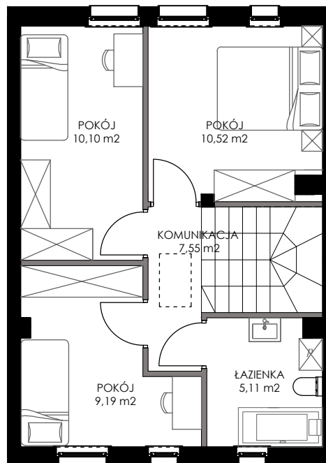
RZUT PIĘTRA
